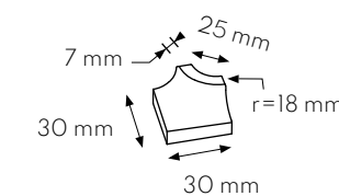
4. PIEDOCA ESTERNO EXTERNAL ELEPHANT'S FOOT 2,5x2,5 . 1"x1"
