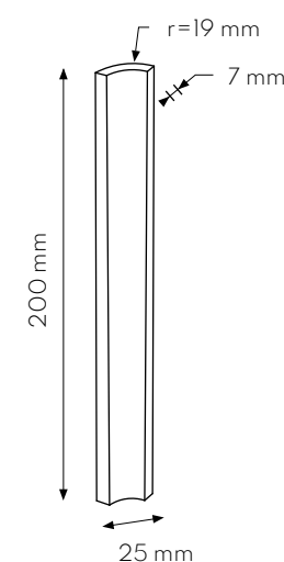
5. CANALETTA INTERNA INTERNAL COVE 2,5x20 . 1"x8"
