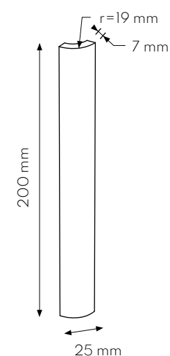
6. CANALETTA ESTERNA EXTERNAL COVE 2,5x20 . 1"x8"
