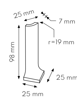
8. ANGOLO ESTERNO EXTERNAL ANGLE 2,5x10 . 1"x4"
