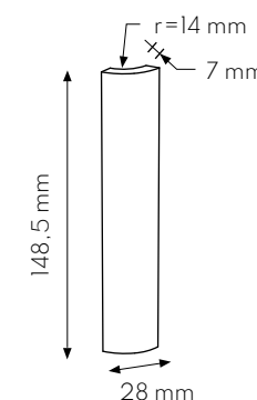
H. CANALETTA ESTERNA 3x15 . 1/4"x6"
