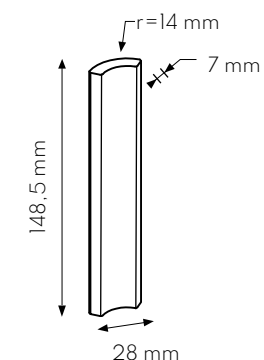
G. CANALETTA INTERNA 3x15 . 1/4"x6"
